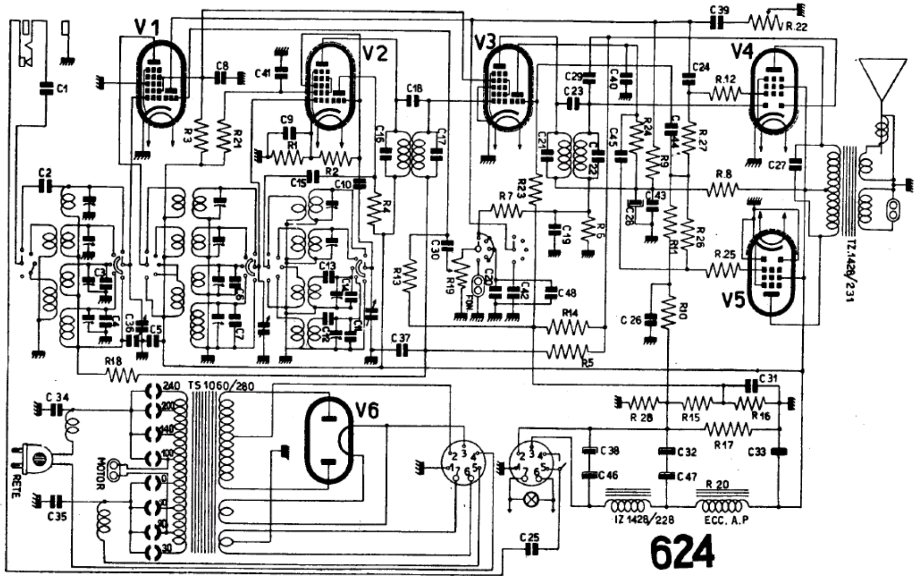
PHONOLA RADIO - Mod. 624 - Gamma onde medie divisa: OM1 da 320 a 600 m, OM2 da 190 a 350 m. Gamma corte da 54 a 25 m, gamma cortissime da 27 a 13 m. Media frequenza 470 kc/s. Potenza d'uscita 7,5 W. Consumo 123 W.
